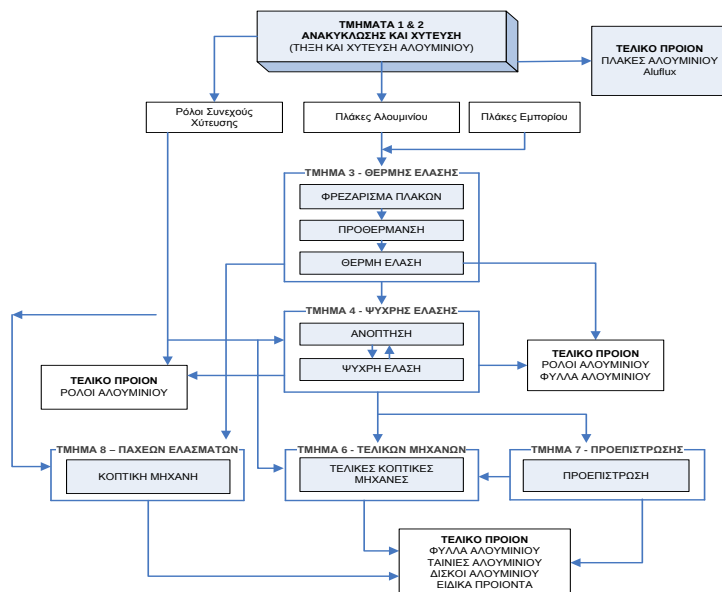
Σχηματική αναπαράσταση των παραγωγικών διεργασιών που συντελούνται στην ΕΛΒΑΛ.
